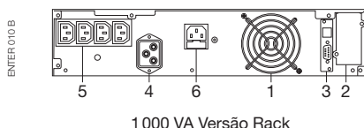
1000 VA Versão Rack
