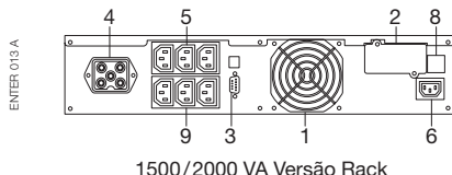
1500/2000 VA Versão Rack
